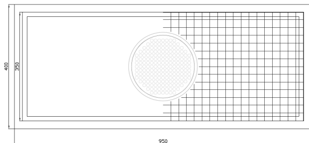
Boven aanzicht
