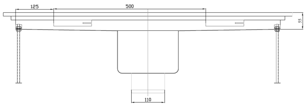
Zij aanzicht
